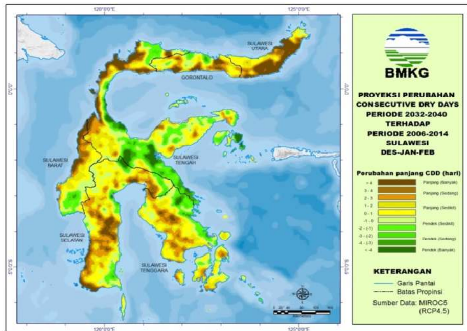
Gambar 2.19 Peta Proyeksi Perubahan Hari Kering Beruntun Periode 2032-2040 di Sulawesi
