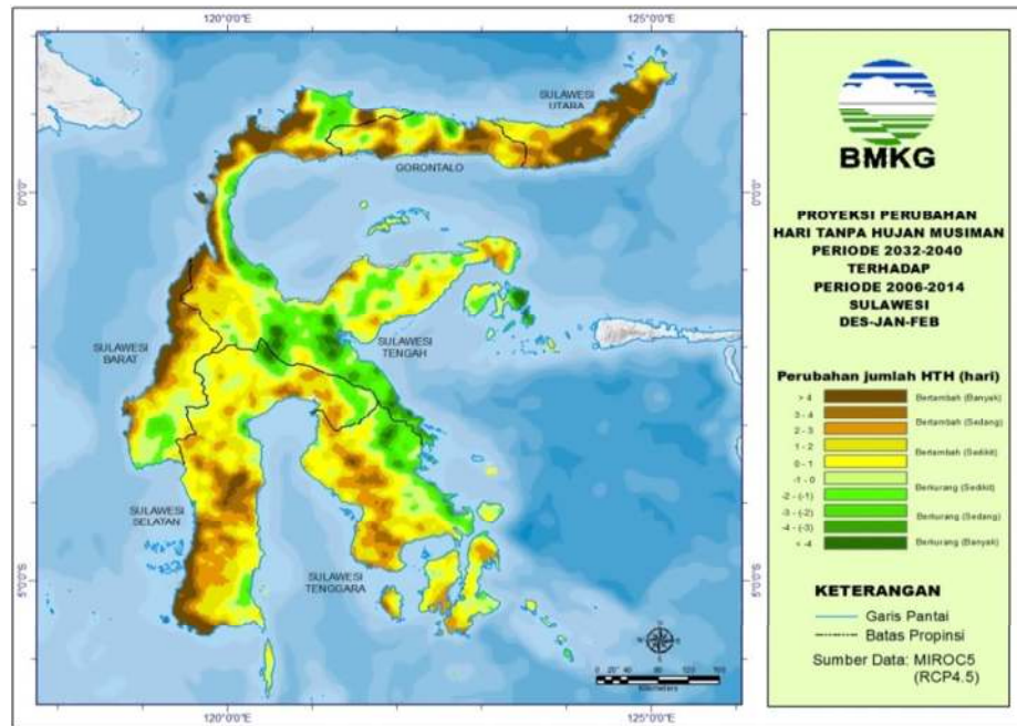
Gambar 2.18 Peta Proyeksi Perubahan Hari Tanpa Hujan Musiman Periode 2032-2040 di Sulawesi
