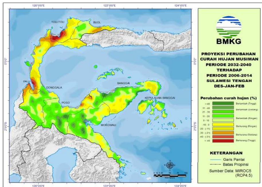
Gambar 2.17 Peta Proyeksi Curah Hujan Musiman Periode 2032- 2040 di Sulawesi
