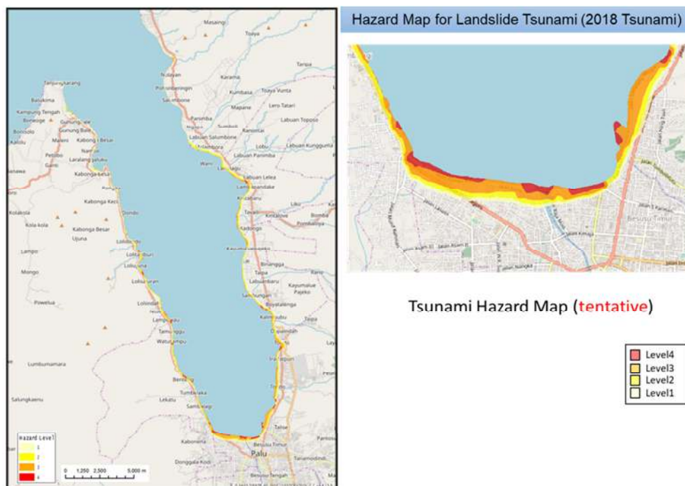
Gambar 2.9 Peta Potensi Tsunami di Kota Palu
