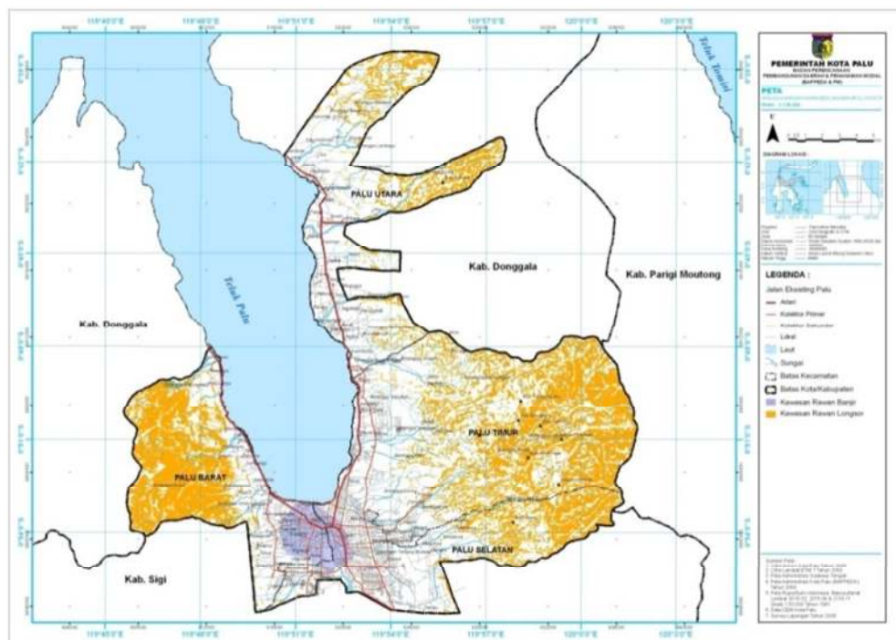
Gambar 2.14 Peta Analisa Rawan Longsor di Kota Palu
