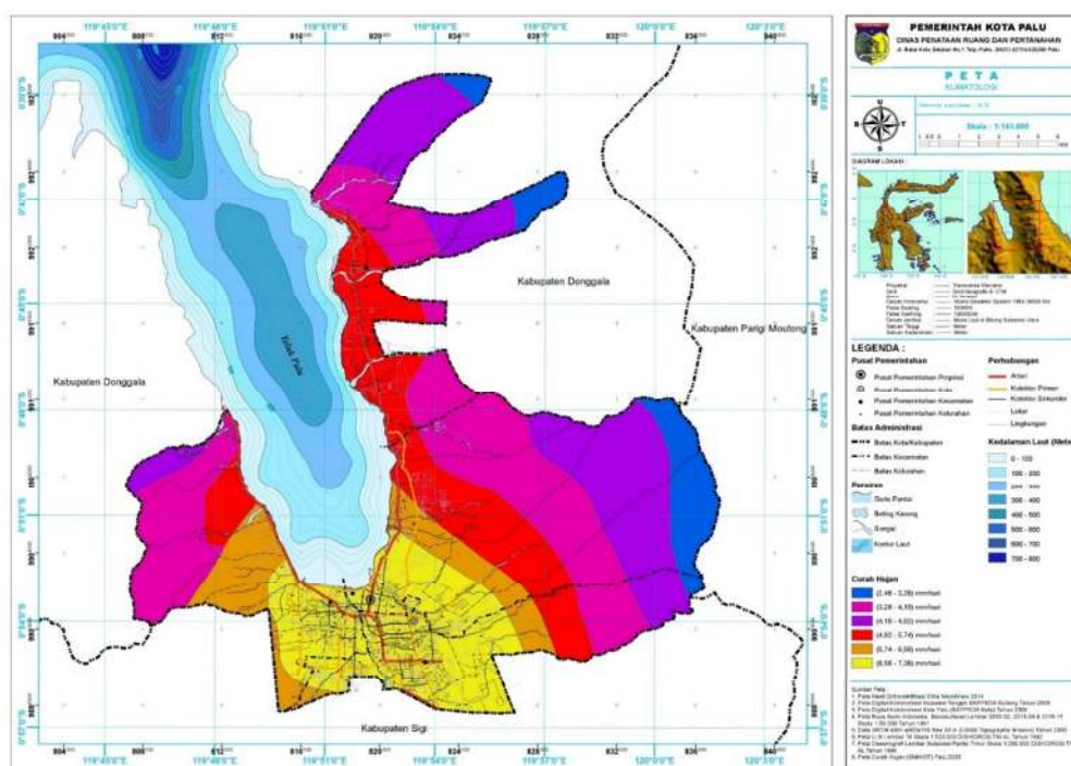
Gambar 2.5 Peta Klimatologi Kota Palu
