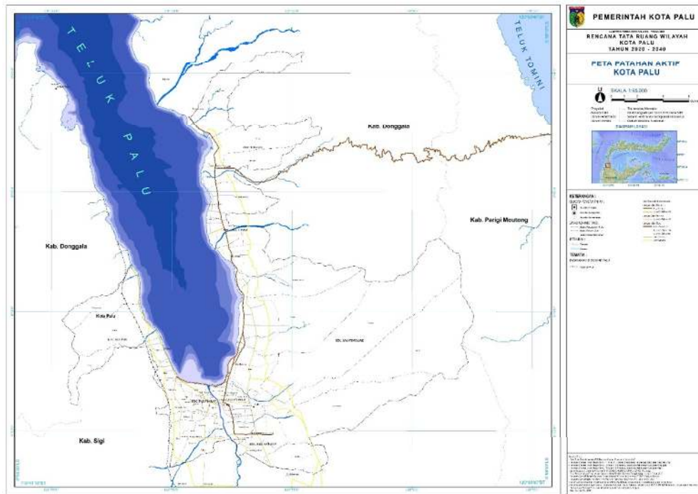
Gambar 2.7 Peta Patahan Aktif di Sekitar Kota Palu
