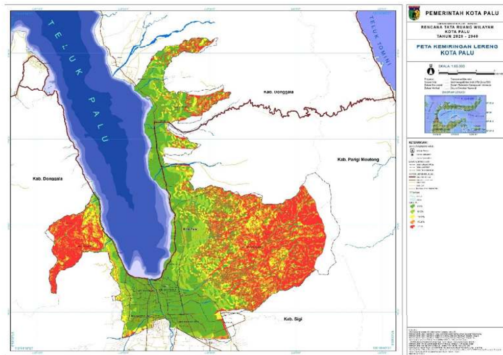
Gambar 2.3 Peta Kemiringan Lereng Kota Palu
