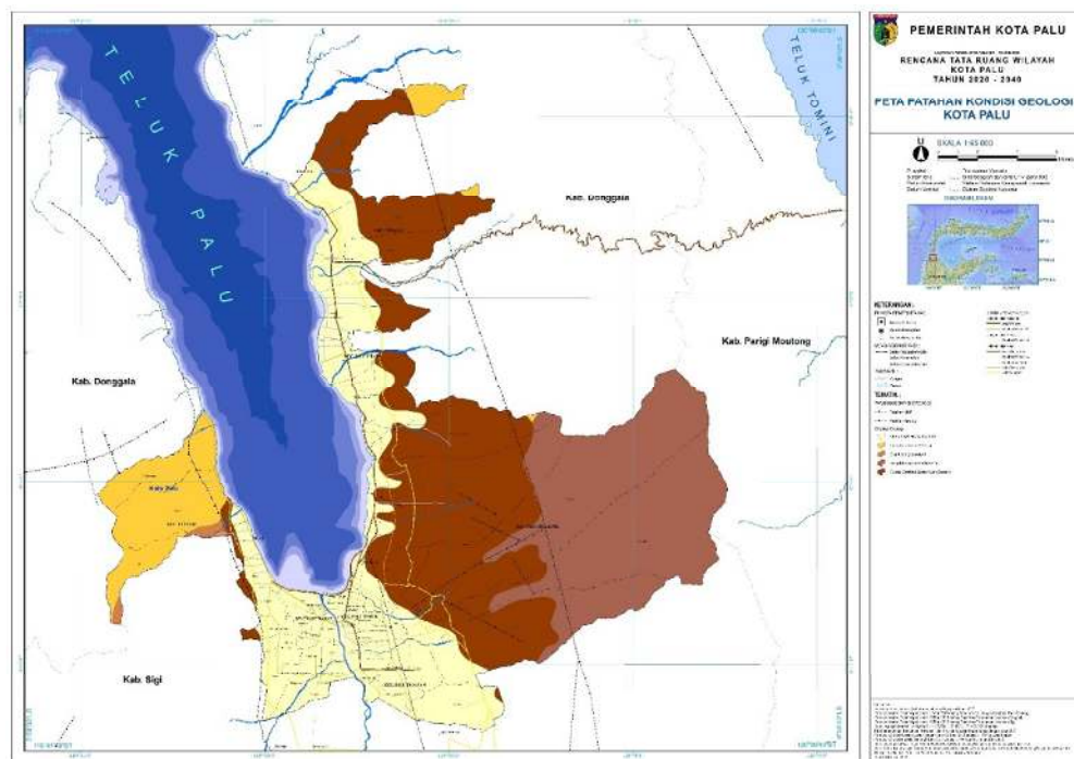
Gambar 2.4 Peta Geologi Kota Palu
